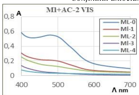
Fig.3. Spectrele de adsorbție în VIS a vinului MI(a), Conținutul antocianilor și O 2 în vin (b)
