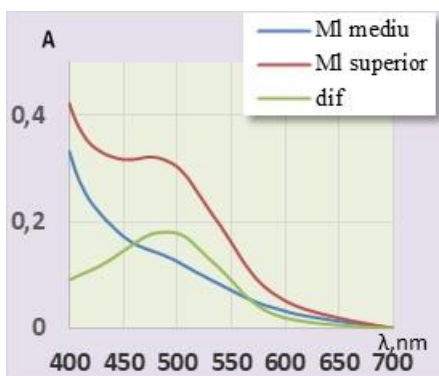
Fig.3. Spectrele de adsorbție în VIS a vinului MI(a), Conținutul antocianilor și O 2 în vin (b)
