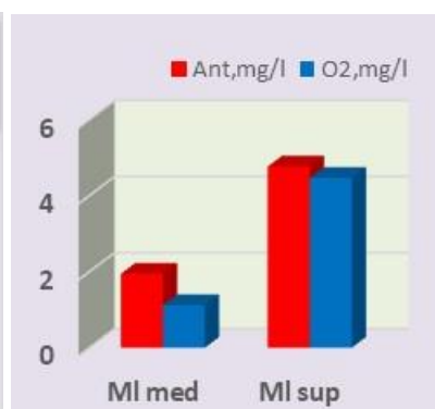
Fig.3. Spectrele de adsorbție în VIS a vinului MI(a), Conținutul antocianilor și O 2 în vin (b)
