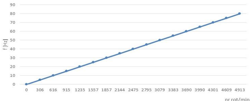
Fig.1. Dependența grafică a turațiilor MEAT de frecvență
