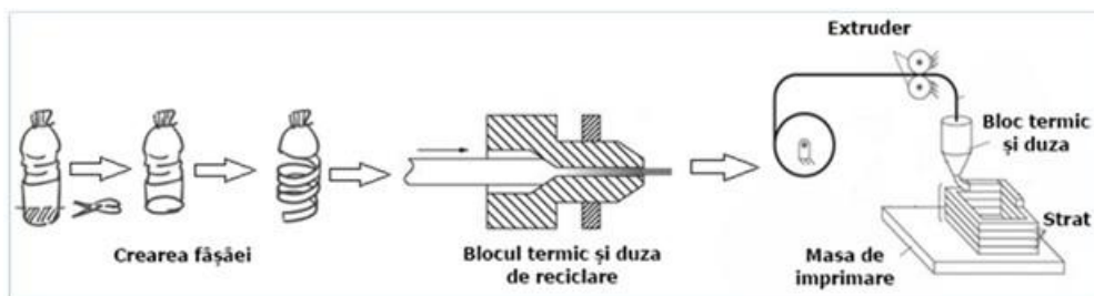
Fig.1. Schema reciclării buteliilor PET cu scopul producției de filament pentru imprimante 3D
