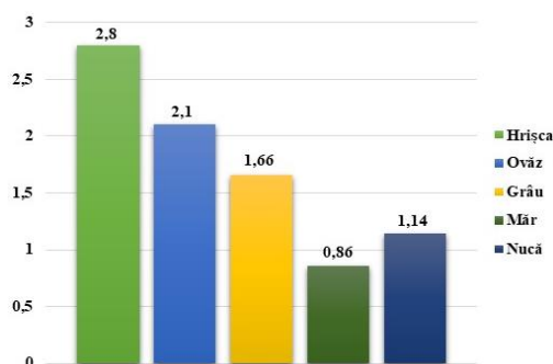
Fig.2. Concentrația Fe^{3+} în produse alimentare, mg/100 g de produs
