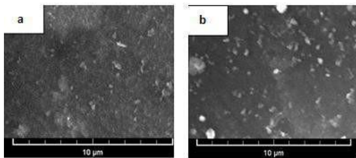
Figura 3. Imaginile SEM a particulelor de compuși ai fierului pe suprafața (a) și în volumul (b) granulelor de polimer de AV-17 după 6 ore de încălzire în apă.
