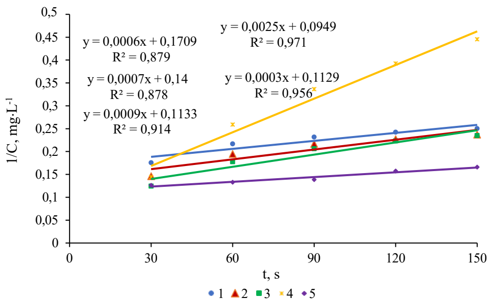
Figura 11. Dependențele \frac{1}{C} = f(t) pentru degradarea CFX în sistemul foto-Fenton la diferite concentrații ale CFX: 1 – 2,0 \cdot 10^{-5} M; 2 – 2,5 \cdot 10^{-5} M; 3 – 3,0 \cdot 10^{-5} M; 4 – 3,5 \cdot 10^{-5} M; 5 – 4,0 \cdot 10^{-5} M
