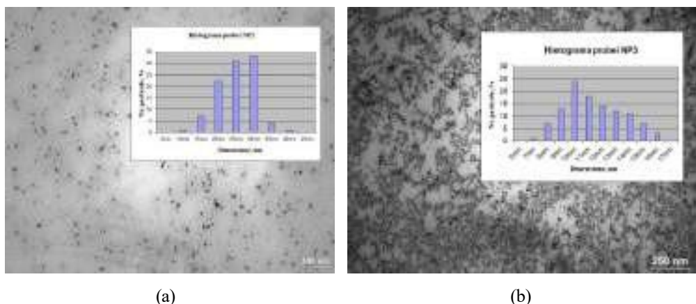
Figura 4. Imagini MET și histogramele distribuției particulelor după dimensiune pentru probele NP2 (a) și NP3 (b)
