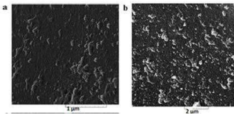
Figura 6. Imaginile SEM a Cr-jarozitului pe suprafața (a) și în volumul granulelor de polimer AV-17.
