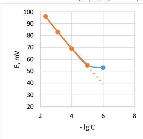
Figura 2. Curba de calibrare pentru EIS 1
