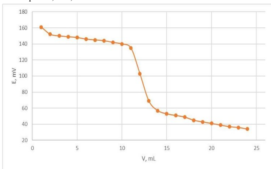
Figura 4. Curba integrală de titrare a soluției model ce conține ioni de zinc cu soluție de hidroxid de sodiu 0,1 mol/L, utilizând în calitate de electrod indicator EIS 2
