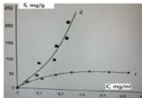
Figura 7. Izoterma sorbției ionilor \text{NO}_2^- pe polimerul Purolite A-400(Cl) (1) și compozitul Purolite A-400 – Cr-jarosit.
