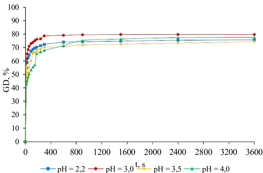
Figura 4. Dependența gradului de degradare a CFX de timp în sistemul Fenton la diferite valori ale pH-ului
