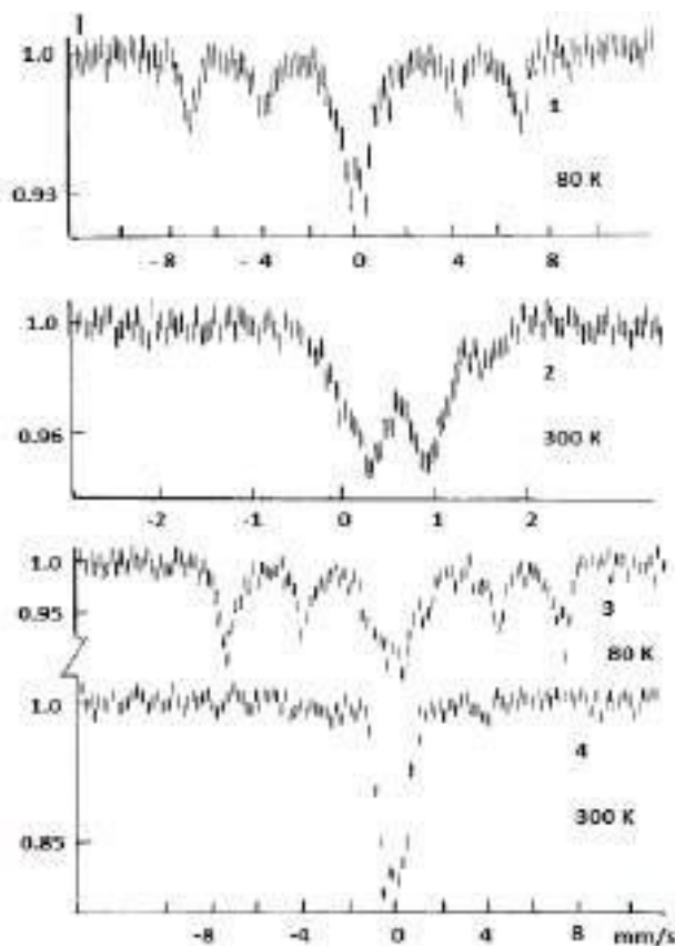
Figura 2. Spectrele Mössbauer a polimerului care conține fier (III) după 3 (pectrele 1 și 2), după 6 (spectrele 3 și 4) cicluri sorbția – fierberea în apă.
