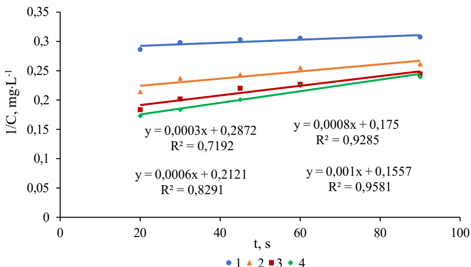
Figura 10. Dependențele \frac{1}{C} = f(C) pentru degradarea CFX în sistemul Fenton la diferite concentrații ale CFX: 1 – 2,0 \cdot 10^{-5} M; 2 – 3,0 \cdot 10^{-5} M; 3 – 3,5 \cdot 10^{-5} M; 4 – 4,0 \cdot 10^{-5} M
