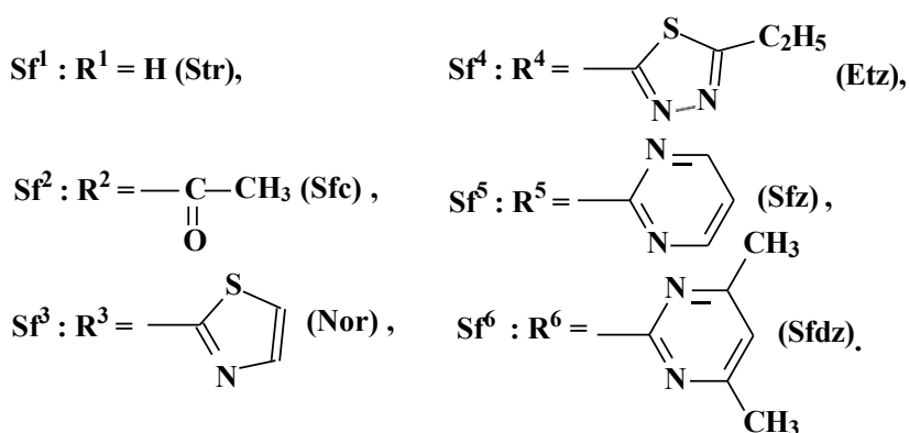
Figura 2. Schema de sinteză a compușilor coordinativi VII-XII
