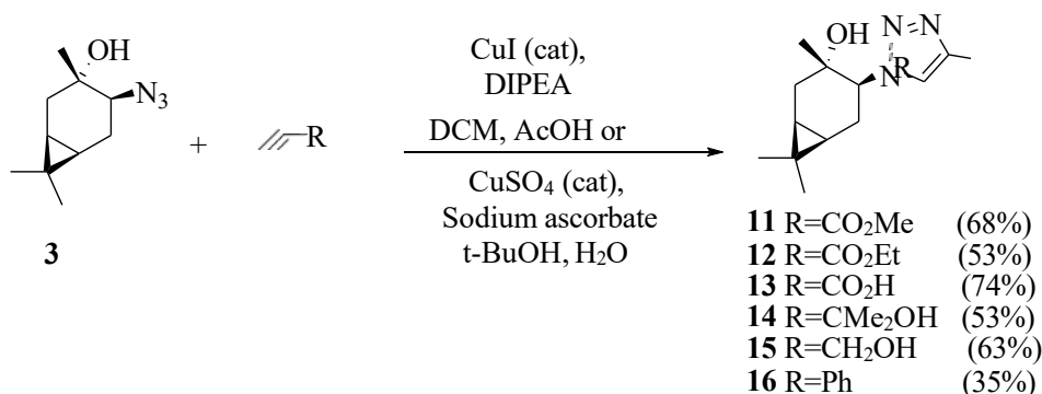
Figura 2. Obținerea 1,2,3-triazolilor din azidoalcoolul 3
