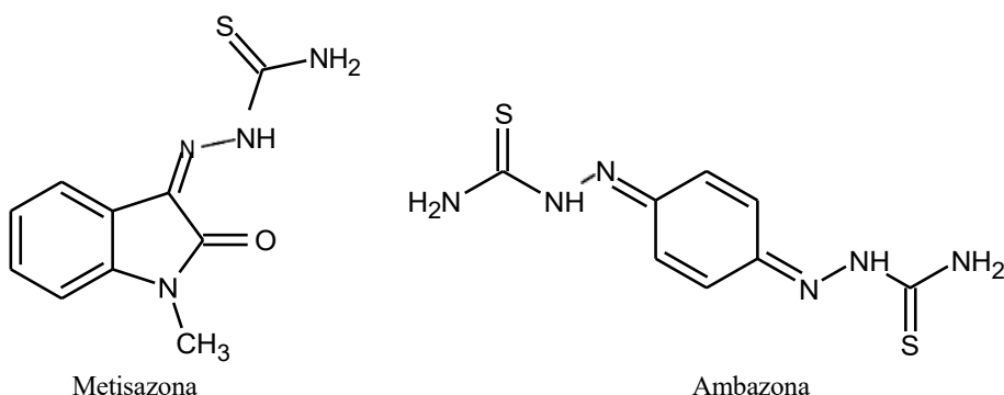
Figura 1. Formule de structură a Metisazonei și Ambazonei
