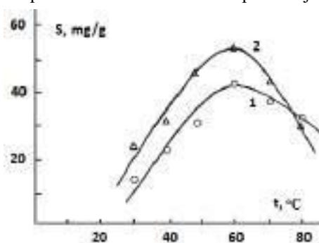
Figura 5. Sobția cationilor care conțin Cr(III) pe polimerii AV-17 (1) și Varion –AD (2) funcție de temperatură.
