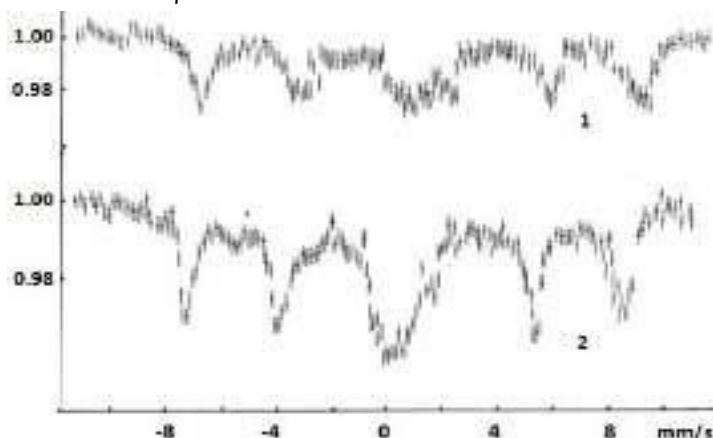
Figura 4. Spectrele Mössbauer obținute la 80 K a copolimerului 4-vinilpiridin: divinilbenzen modificat cu acid monocloracetici (1) și acid acrilic (2) care au reținut \text{Fe}^{3+} din soluția de \text{Fe}_2(\text{SO}_4)_3 după 3 cicluri sorbția-fierberea în apă.
