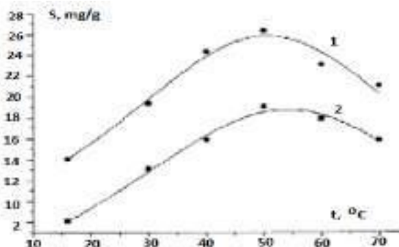
Figura 1. Sorbția ionilor de Fe^{3+} pe polimerii AV-17x8 și Varion-AD funcție de temperatură.
