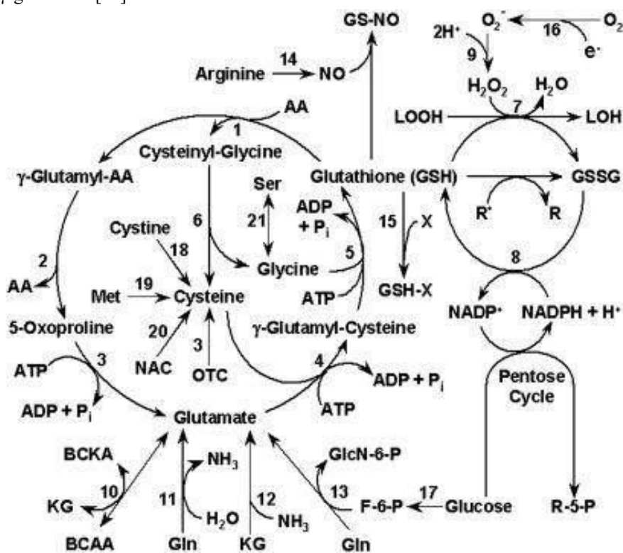
Figura 1. Metabolismul glutationului [1].
