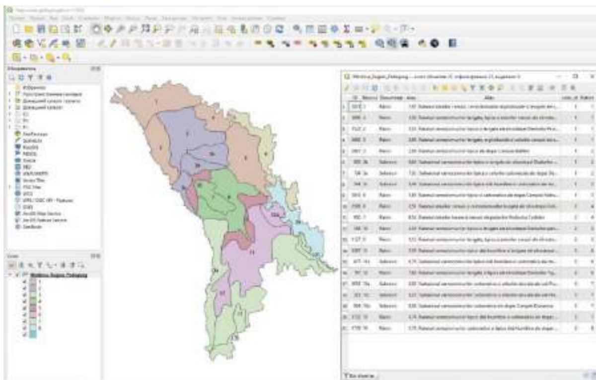
Figura 4. Regionarea pedogeografică
