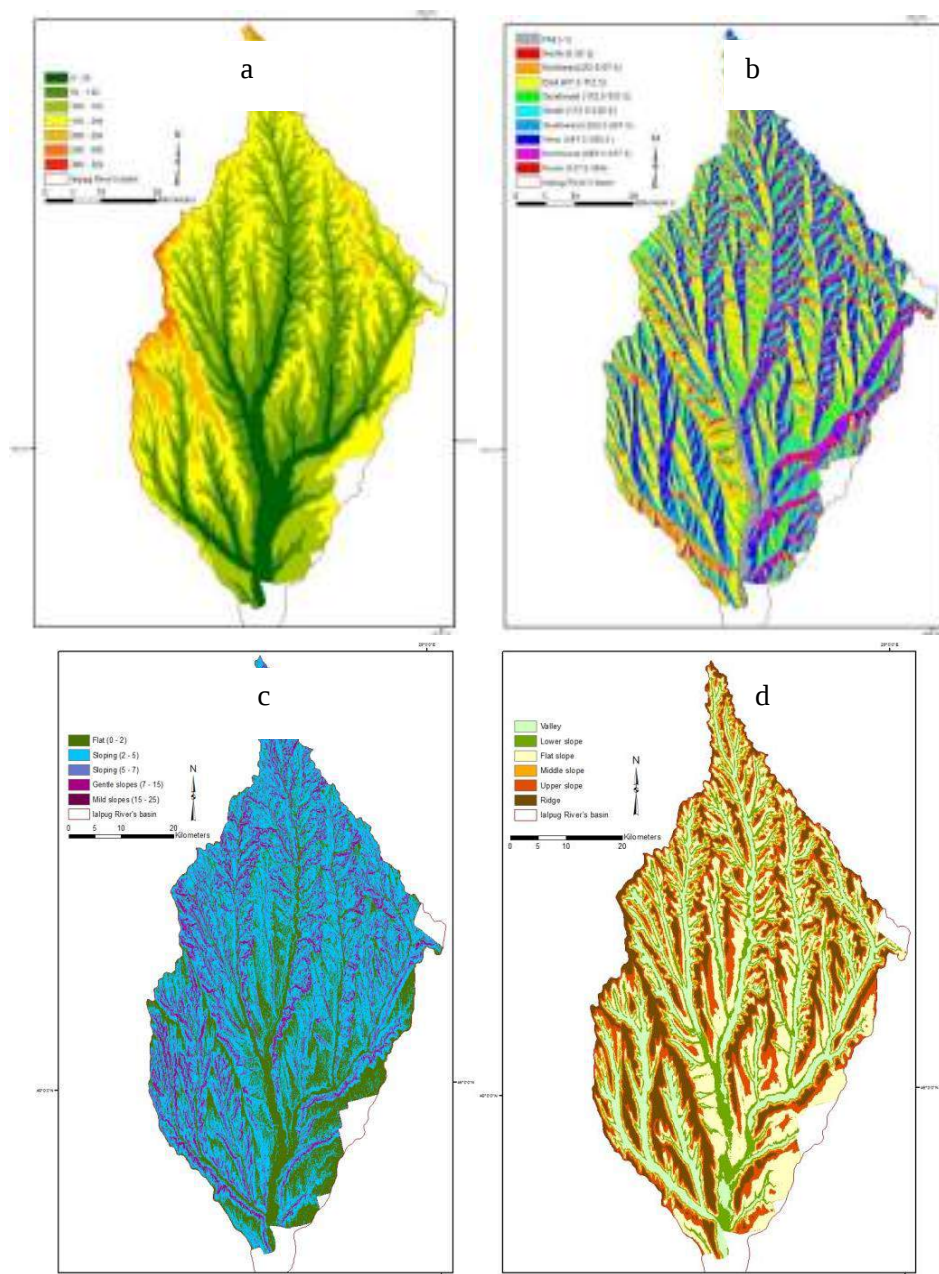
Fig. 1. (a) Elevation, (b) Aspect, (c) Slope (°), (d) TPI.
