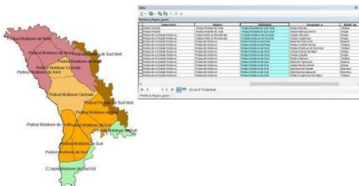
Figura 2. Subregiuni geomorfologice
