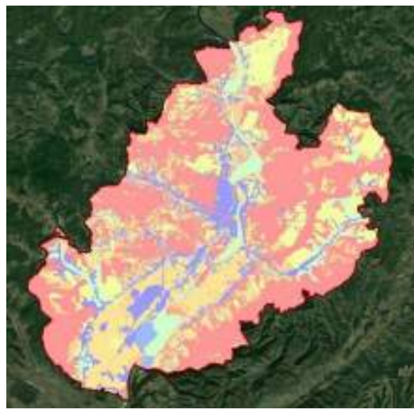
Fig. 6. Harta rasterului de rezistență la mișcare prin peisajul zonei de studiu
