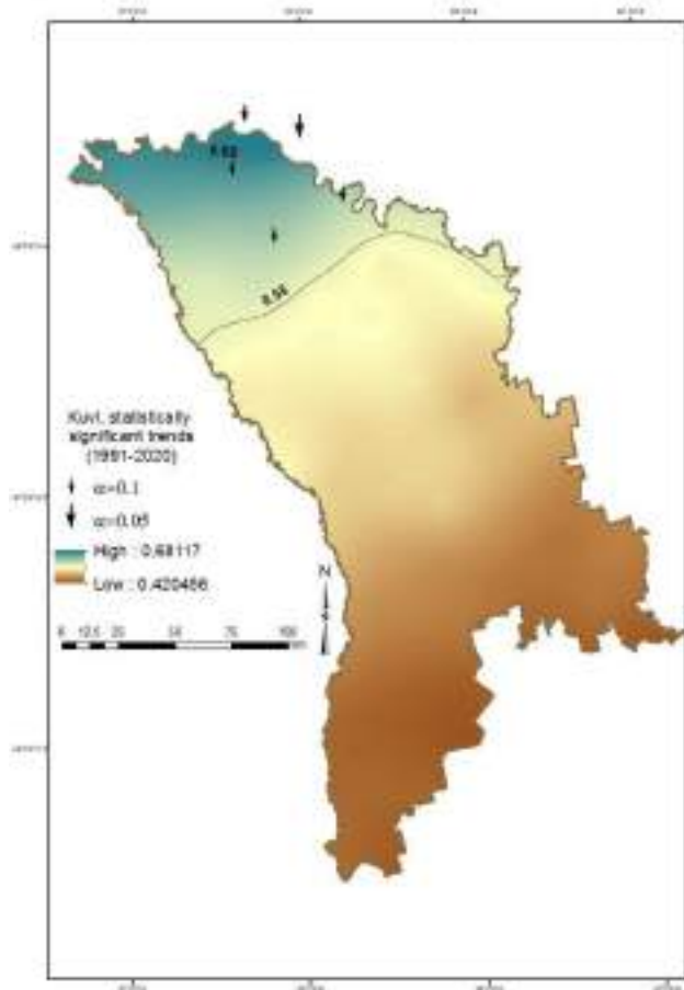
Fig.2. Interpolarea prin kriging a indicelui de umiditate Kuvl
