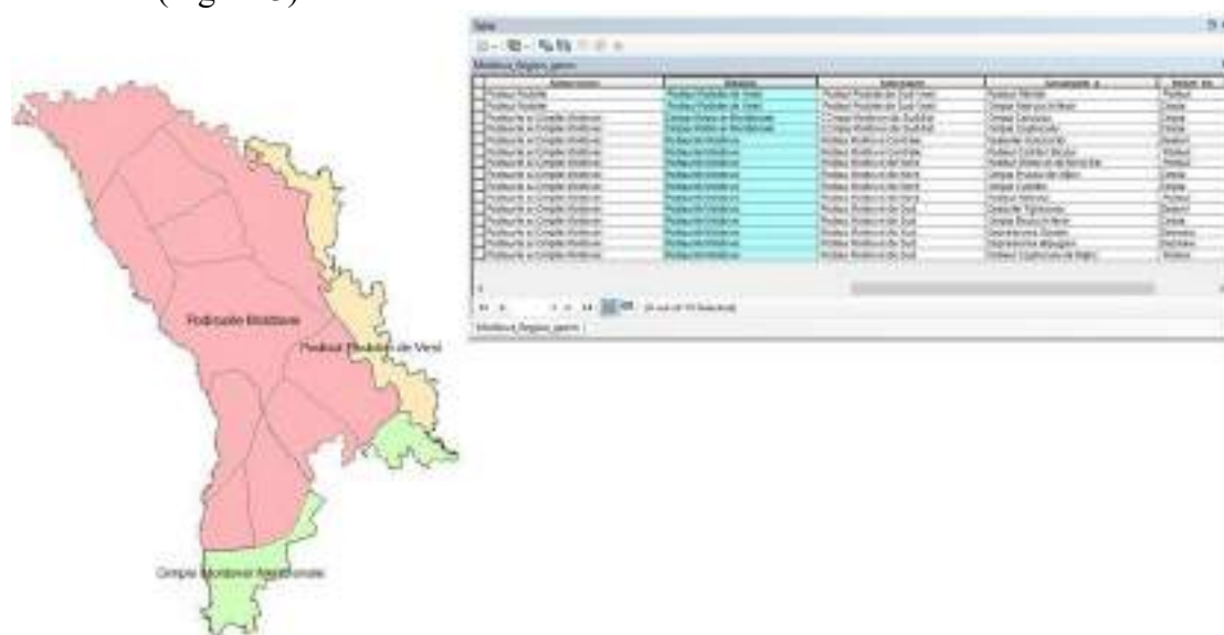
Figura 3. Regionarea geomorfologică
